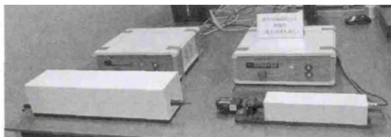
图 8 激光纳米测尺
