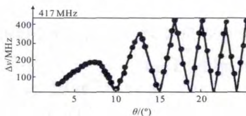
图 3 激光频率分裂随石英片旋转角度变化
