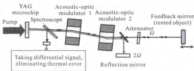
(a) 激光回馈干涉仪原理图
