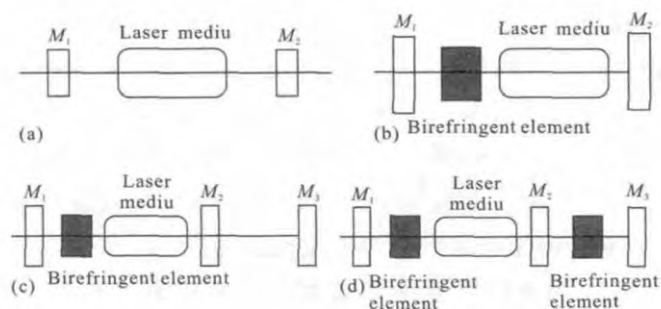
图 1 不同激光腔结构
