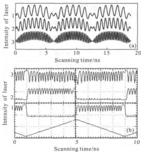
图 5 非准直外腔调谐时两正交偏振激光的光强曲线
