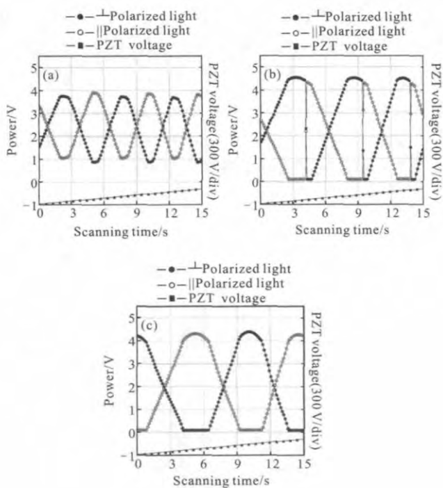
图 4 激光谐振腔调谐时两正交偏振光光强曲线
